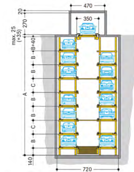
PARKING AUTOMATYCZNY PRZEKRÓJ OK. 8 POZIOMÓW, 14 MIEJSC POSTOJOWYCH
